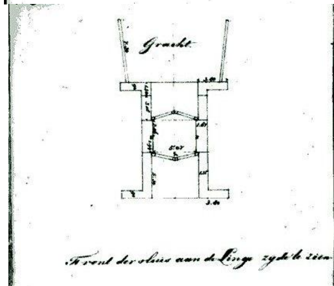
Afb.15 Dwarsdoorsnede van de sluis Oostgracht/Linge en plattegrond van de sluis in 1830. Uit Schetsboekje van Ir. L.J.A. van der Kun
