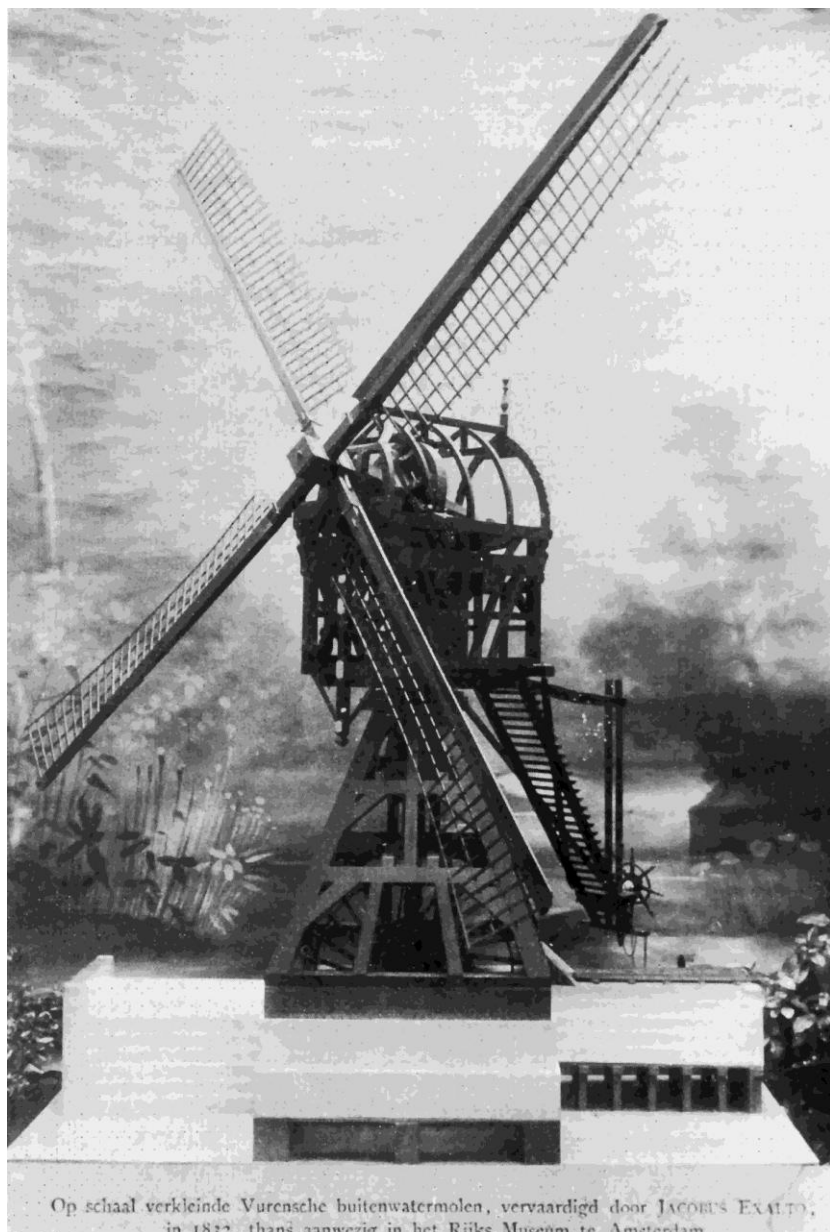
Afb.2a Op schaal verkleinde Vurense voormolen in de Hondswaard, vervaardigd door de molenbouwer Jacobus Exalto in 1832 (Rijksmuseum)
